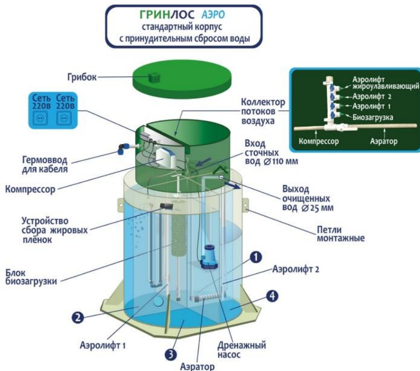
Рисунок 2. Схема модели с принудительным сбросом сточных вод и стандартным корпусом
